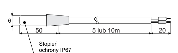
Rys.4. Wymiary czujnika przewodowego.
