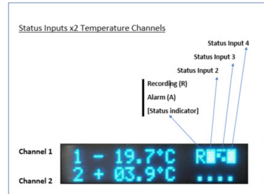
Rysunek 1.4.1 Wyświetlacz Wejścia Statusowe x2 Kanały Temperatury
